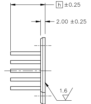
MATERIAL : A6063 FINISH : BLACK ANODIZE DIMENSIONS : mm
